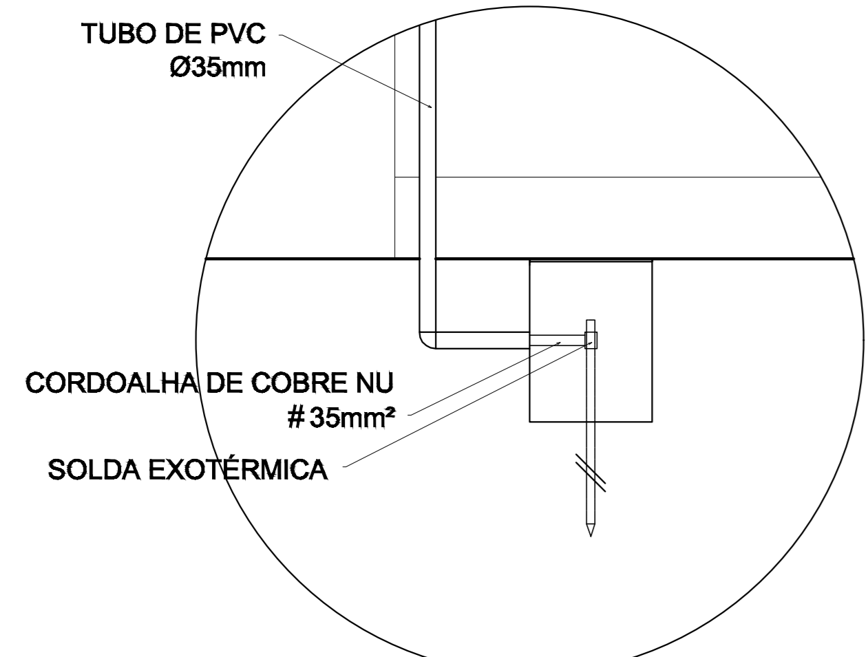
DET. CAIXA INSPEÇÃO
