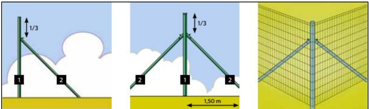
Figura 03 – Detalhes dos postes da barreira física
