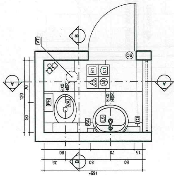
I.S. CONS. GINECOLÓGICO PLANTA
